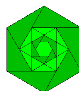
hata 3 100 2
