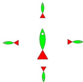
halraj 100 2 4
