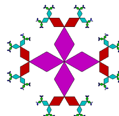
növény 5 30
