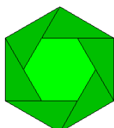
hata 1 100 2
