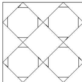
négyzetek 2 200
