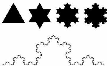
Koch farktál
