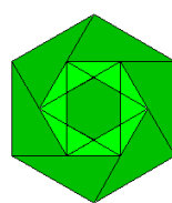
hata 2 100 2
