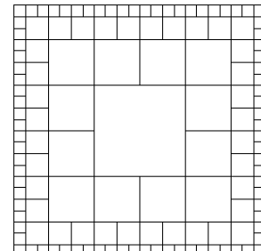
négy 4 100
