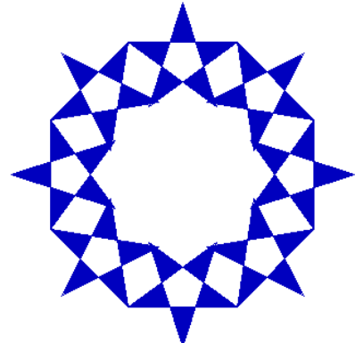
csillagok 8 100
