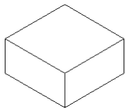
HATA 50 100
