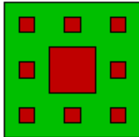
sier 2 100
