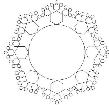
csipke 100 3
