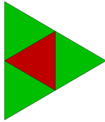
sier 1 100
