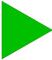
sier 0 100
