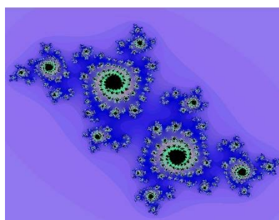
Júlia halmaz
