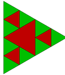
sier 2 100
